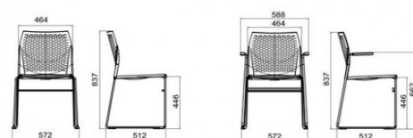
DIMENSIONI - DIMENSIONS
